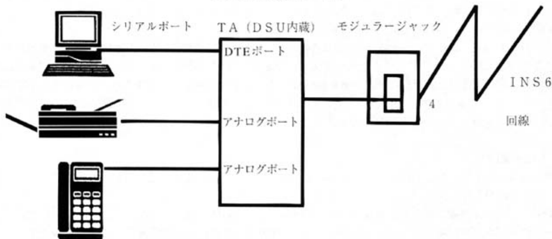
～ISDN接続イメージ図～
